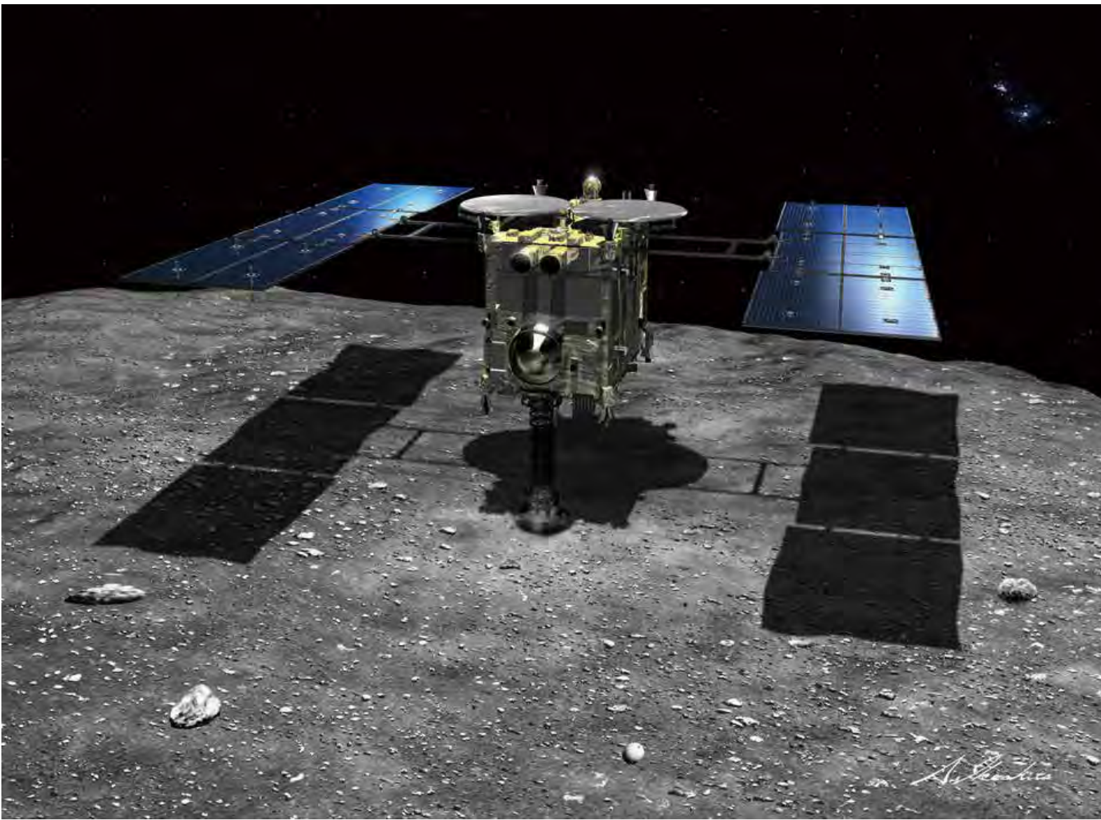
小惑星表面にタッチダウンする「はやぶさ2」の想像図 ©池下章裕
